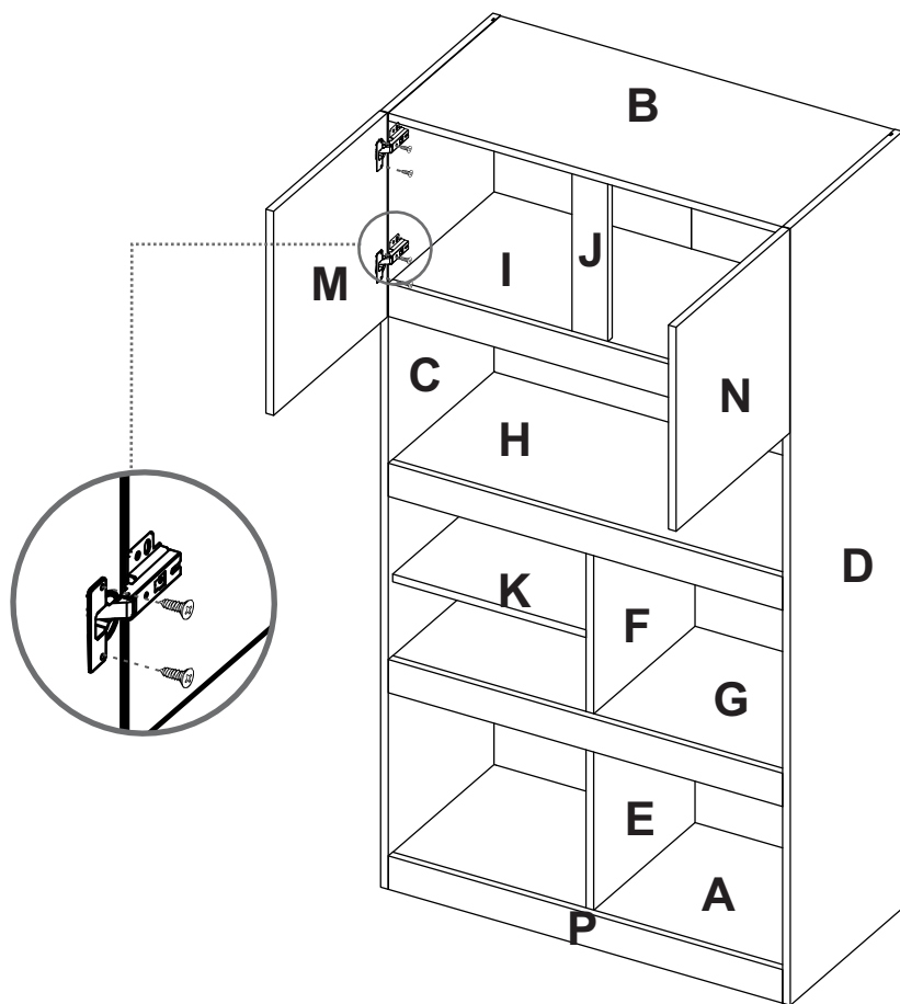
AJUSTE DE PROFUNDIDAD / DEPTH ADJUSTMENT
