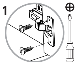
1 Ajuste de las bisagras Hinge adjustment
