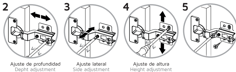
Ajuste de las bisagras Hinge adjustment
