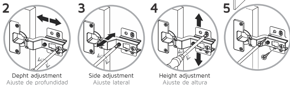
Ajuste de las bisagras Hinge adjustment
