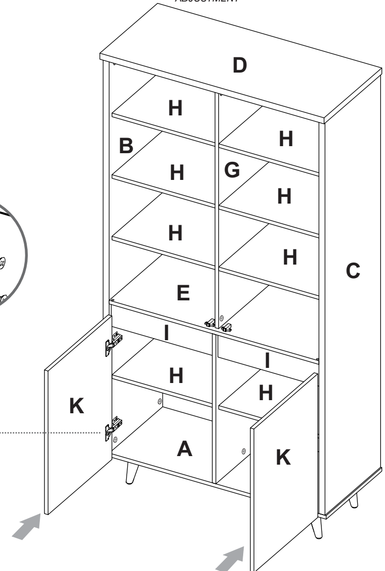
AJUSTE DE PROFUNDIDAD / DEPTH ADJUSTMENT
