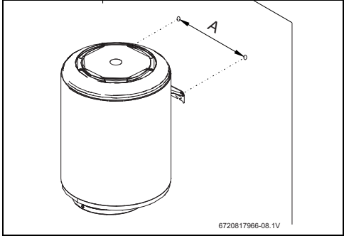
Fig. 7 Instalación en posición vertical
