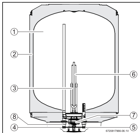
Fig. 4 Estructura
